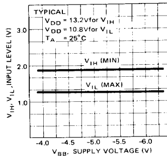
V IH , V IL INPUT LEVELS vs V BB SUPPLY VOLTAGE
