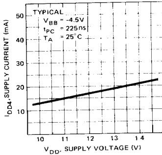
I DD4 (PAGE-MODE) vs V DD SUPPLY VOLTAGE
